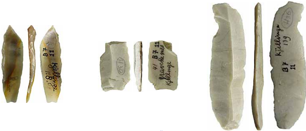
Afb. 3 Terugggevonden artefacten van De Kjellingen (Frl.). Van links naar rechts: een kleine Tjongerspits, een mogelijk Tjongerspits-fragment en een kling met kerf en geretoucheerde top (ware grootte; bijlage II nrs. 9, 6 en 9)
